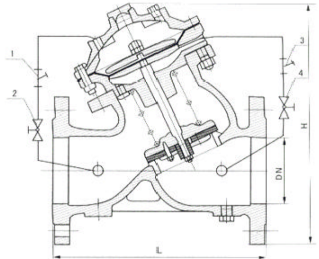
1、过滤器 2、小球阀 3、过滤器 4、小球阀
