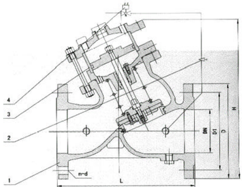
1、阀体 2、针阀 3、缸套 4、电磁阀
