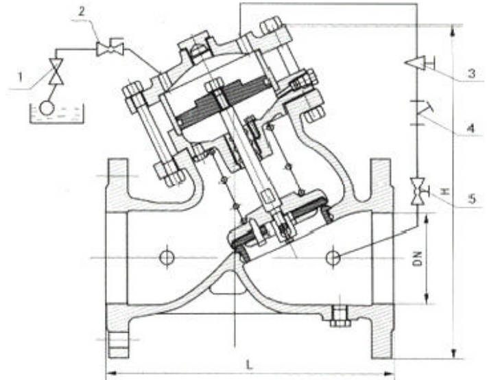
1、小浮球阀 2、小球阀 3、针型阀 4、过滤器 5、小球阀
