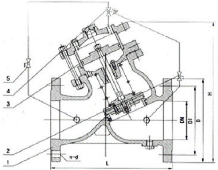
1、阀体 2、球阀 3、缸套 4、导阀 5、球阀
