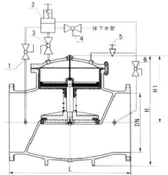
1、小球阀 2、导阀 3、小球阀 4、小球阀 5、针形阀 6、小球阀
