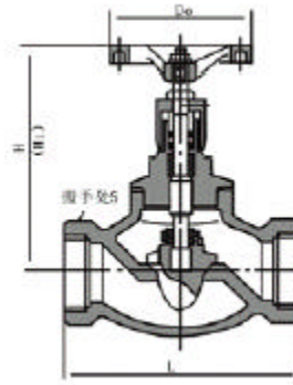
内螺纹连接自锁手动调节阀 (TJ10H 型)
