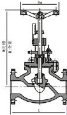
法兰连接手动调节阀 (TJ40H 型)
