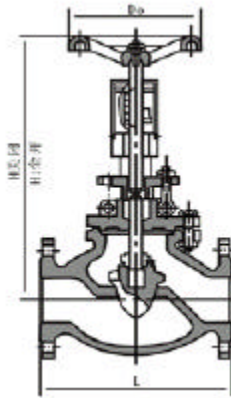
法兰连接自锁手动调节阀 (TS40H 型)
