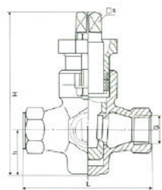
X14W-1.0 三通铸铁内螺纹旋塞阀
