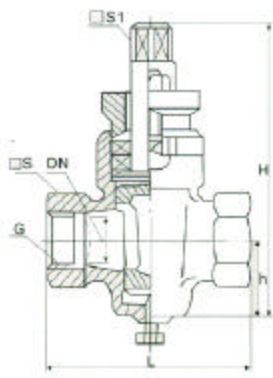
X13W-1.0 二通内螺铸铁旋塞阀
