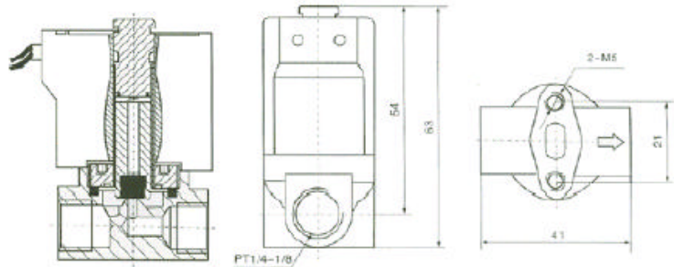
RSSM 外形尺寸结构图
