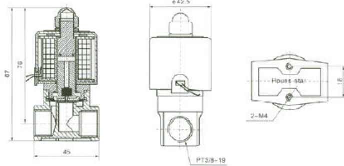
UD-C 外形尺寸结构图
