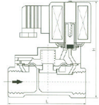
结构示意图 (常闭式)
