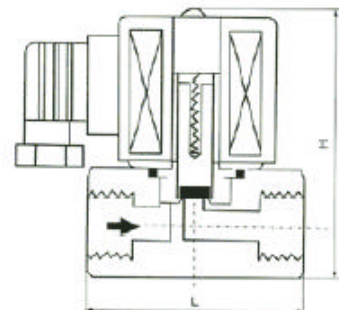
3- 6 直动式结构示意图
