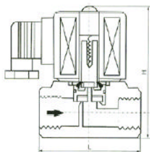
15- 25 分步直动式结构示意图
