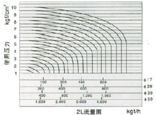
2L流量图 kg/h
