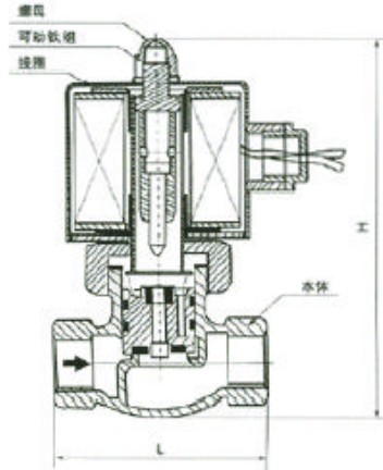
内部结构外形示意图
