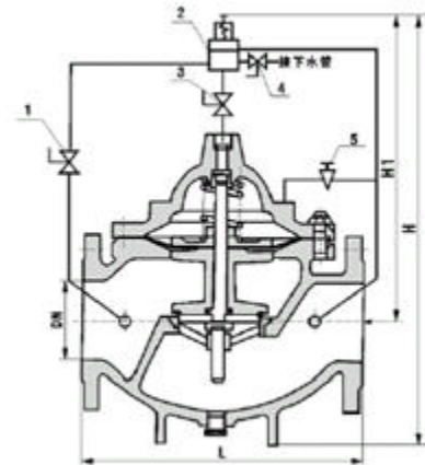
1、小球阀 2、导阀 3、小球阀 4、小球阀 5、针形阀
