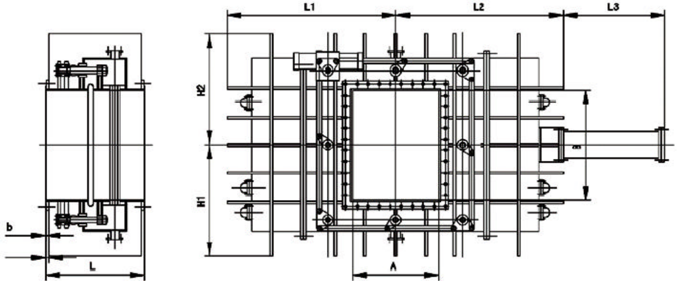
BYCZ F 749 型液动(方形)封闭式眼镜阀外形尺寸
