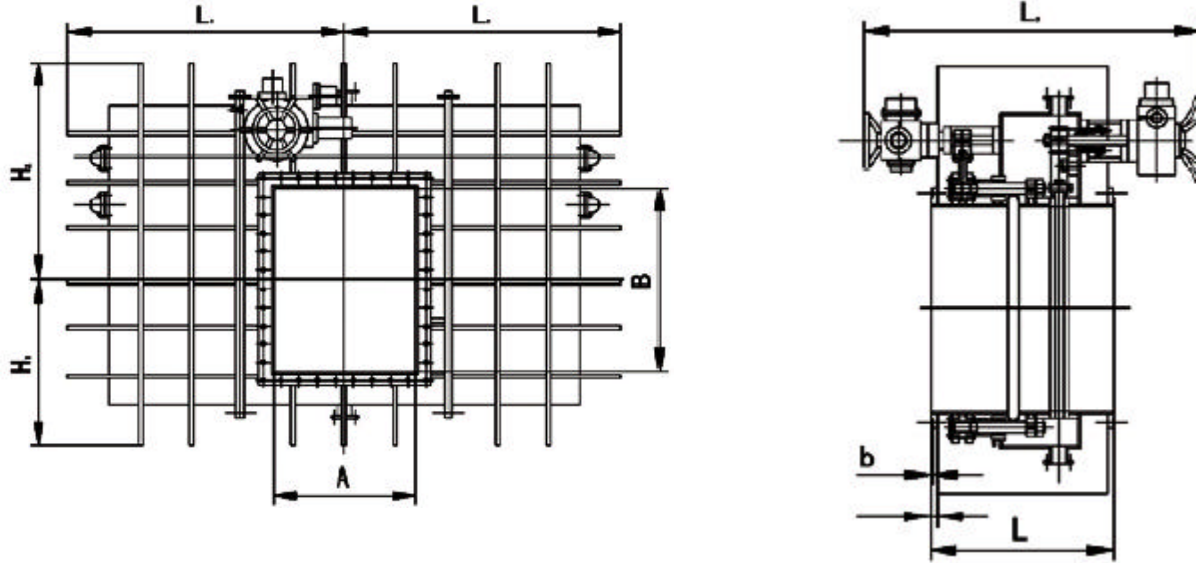
BYCZ F 949 型电动(方形)封闭式眼镜阀外形尺寸
