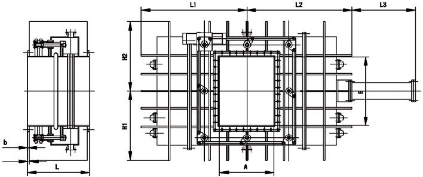
BYCZ F 649 型气动(方形)封闭式眼镜阀外形尺寸
