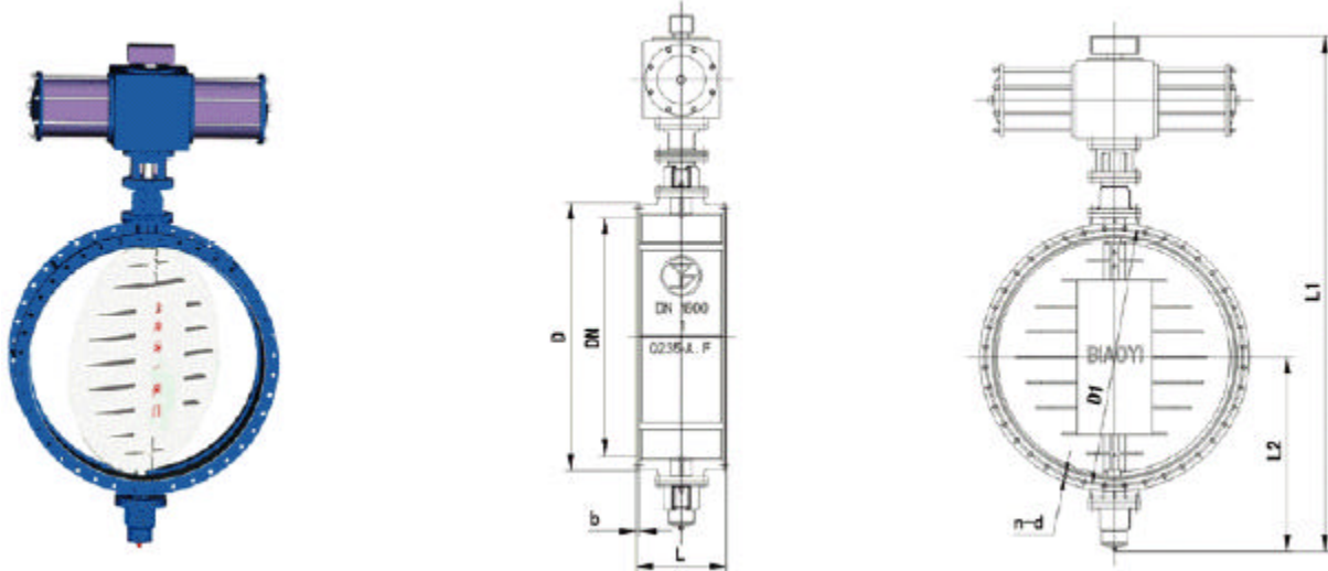
RMTD641W 气动通风蝶阀主要外形连接尺寸
