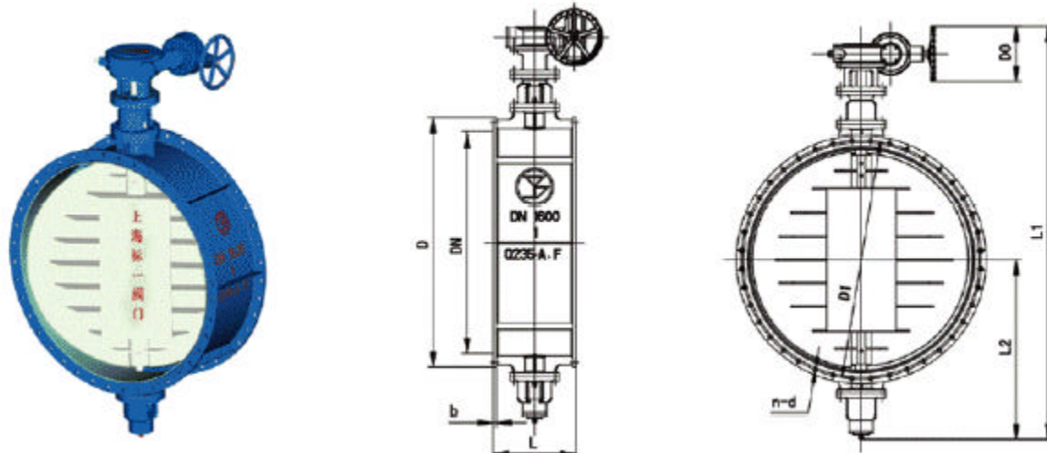
RMTD341W 涡轮传动通风蝶阀主要外形连接尺寸
