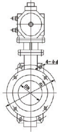
RMD673H-10/16 气动对夹式硬密封蝶阀主要外形连接尺寸
