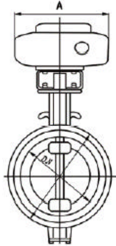
RMWBEX (D972X) -6/10/16 电动对夹式软密封蝶阀主要外形连接尺寸
