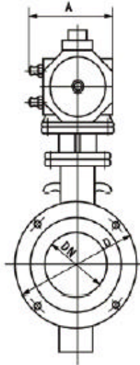
RMWBPX (D672X) -6/10/16 气动对夹式软密封蝶阀主要外形连接尺寸
