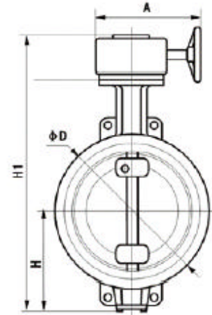
蜗轮型蝶阀
