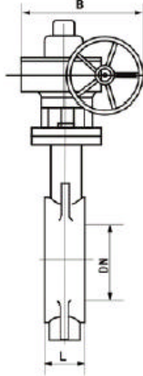
RMD971X-6/10/16 对夹式电动软密封蝶阀主要外形连接尺寸
