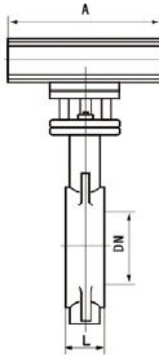
RMD671X-6/10/16 对夹式气动软密封蝶阀主要外形连接尺寸
