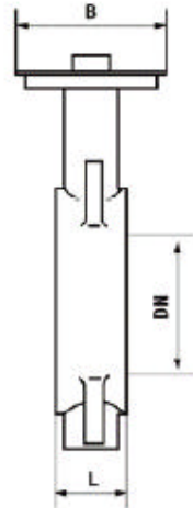
RMD71X-6/10/16 对夹式软密封蝶阀主要外形连接尺寸
