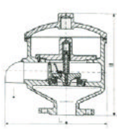
HX5型单呼阀 DN50-250
