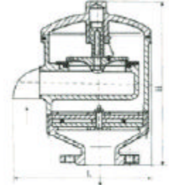
HXF6型阻火单吸阀 DN50-250
