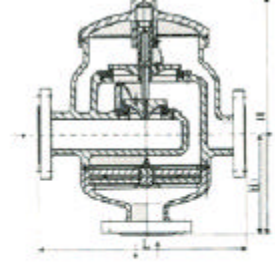
HXF2型带双接管阻火呼吸阀 DN50-250
