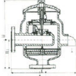
HXF3型带吸入接管阻火呼吸阀 DN50-250
