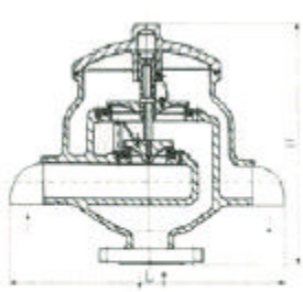
HX1型呼吸阀 DN50-400
