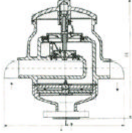
HXF1型阻火呼吸阀 DN50-400
