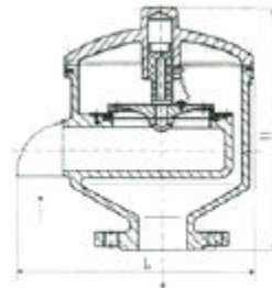
HX6型单吸阀 DN50-250
