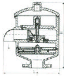
HXF5型阻火单呼阀 DN50-500
