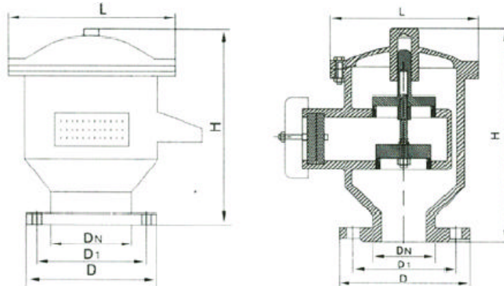
结构示意图
