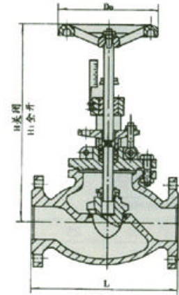
法兰连接手动调节阀(TJ40H型)
