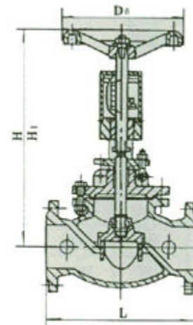
KPF-16型平衡阀
